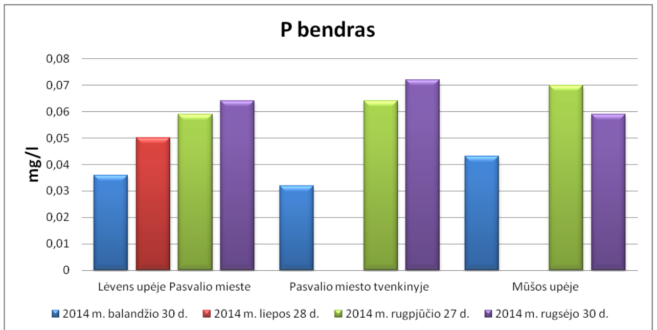
20 pav. Pasvalio rajono savivaldybės paviršinio vandens P bendrojo tyrimo rezultatų vizualizacija.
