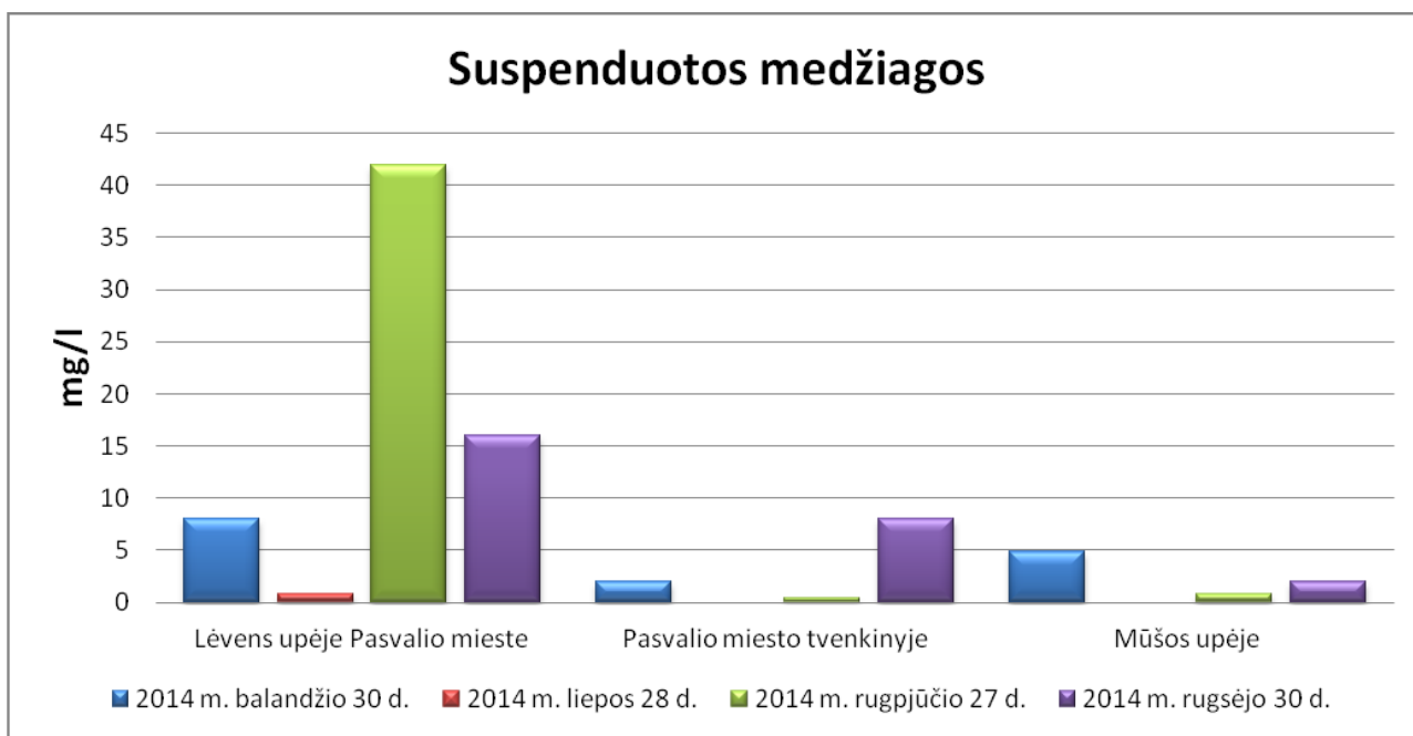
24 pav. Pasvalio rajono savivaldybės paviršinio vandens Suspendingtų medžiagų tyrimo rezultatų vizualizacija.
