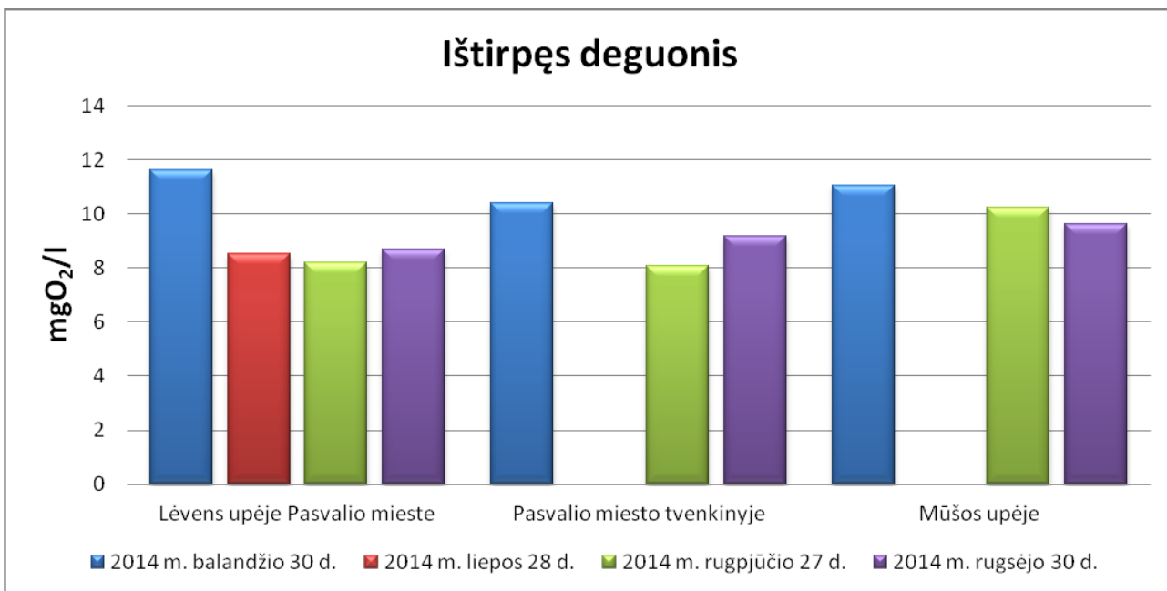
22 pav. Pasvalio rajono savivaldybės paviršinio vandens Ištirpęso deguonies tyrimo rezultatų vizualizacija.
