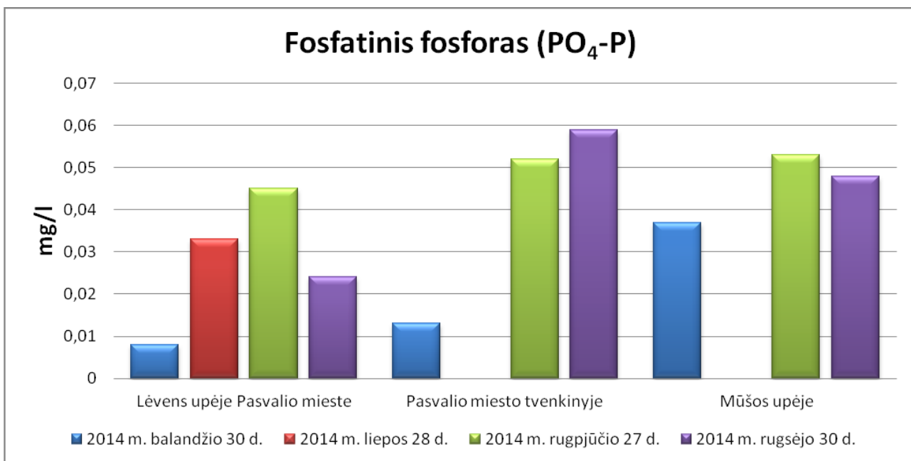
21 pav. Pasvalio rajono savivaldybės paviršinio vandens Fosfatinio fosforo (PO 4 -P) tyrimo rezultatų vizualizacija.
